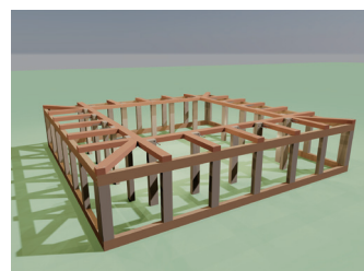
16 內柱角
