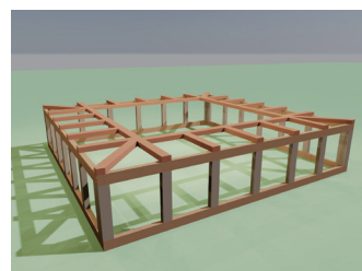
15 椅面框架組立
