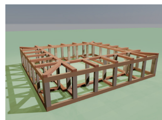
20 底框完成
