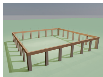
06 鎖其餘柱腳
