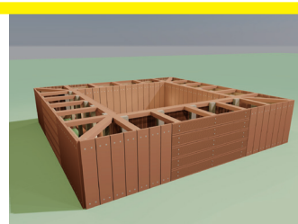
27 四周封板完成
