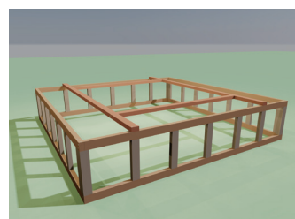
10 主內框架完成
