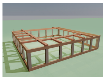
11 架 - 左前框架
