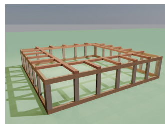
13 鎖 - 右後框架
