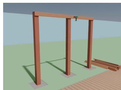
14 依序引洞鎖螺絲
