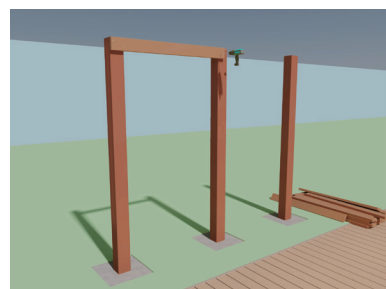
13 橫樑 + 鎖螺絲
