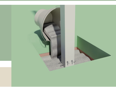
A03 固定
