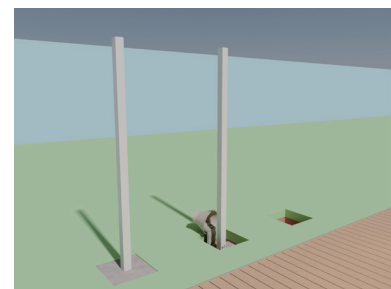
06 倒混凝土固定
