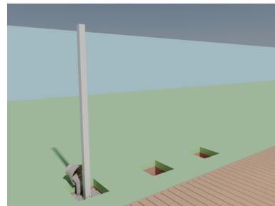
04 倒混凝土固定
