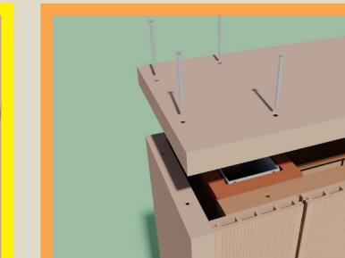
E 上封板鎖螺絲
