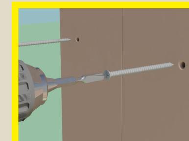
D01 側封板引洞
