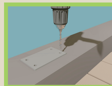
A 電鑽引洞
