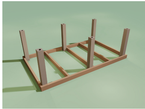
05 桌腳上螺絲
