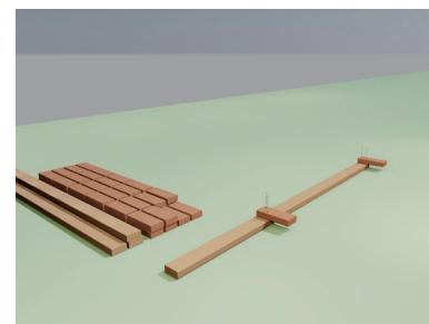
02 組立柱
