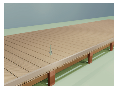
13 收邊條
