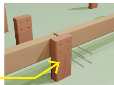
立柱引 4 洞
