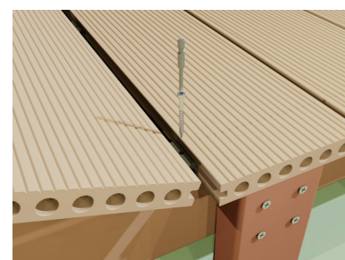
09 使用起子頭
